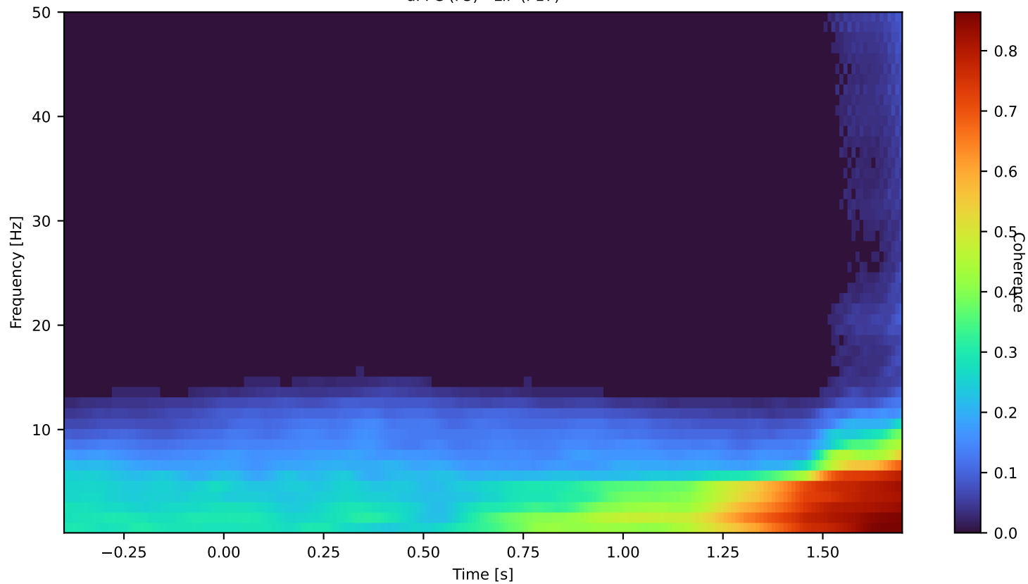
dPFC (F5) - LIP (P17)
